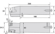
Right Hand Toolholder 69 391 431 10
